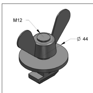
MODFRAME® FixBOB
