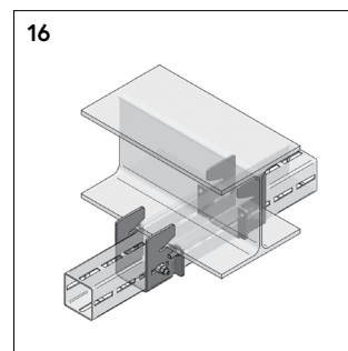
MODFRAME® Clamping shoe
