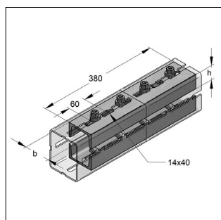
MODFRAME® Connector
